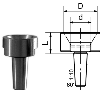
Kegelgöbe / Sklon kuželu
