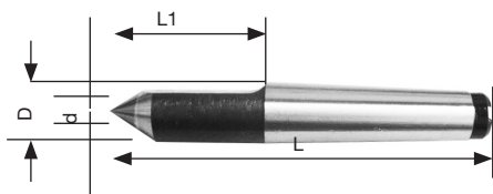
Hartmetalleinsatz mit verlängerter halber Spitze Prodloužený poloviční karbidový hrot
