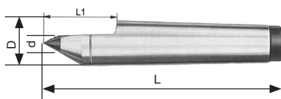
Hartmetalleinsatz mit halber Spitze Poloviční karbidový hrot
