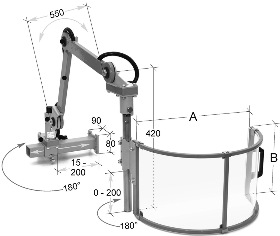
Abb. zeigt Befestigung von links Obrázek ukazuje montáž zleva
